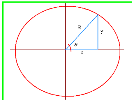
CIRCUNFERENCIA UNIDAD (R=1)
