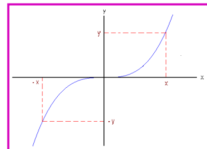
Simetría respecto al origen
