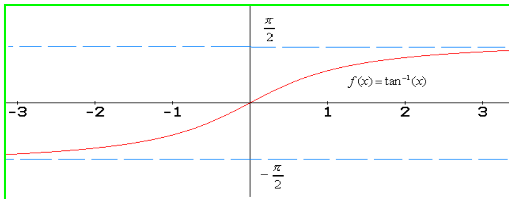
Función Tangente Inversa
